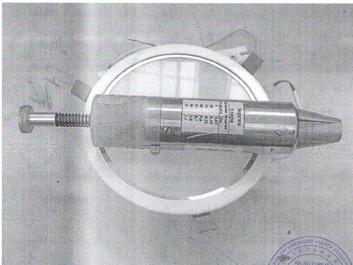
Рис. 1 Вид на испытательное пружинное ударное устройство ИПУУ-2 перед испытаниями.
