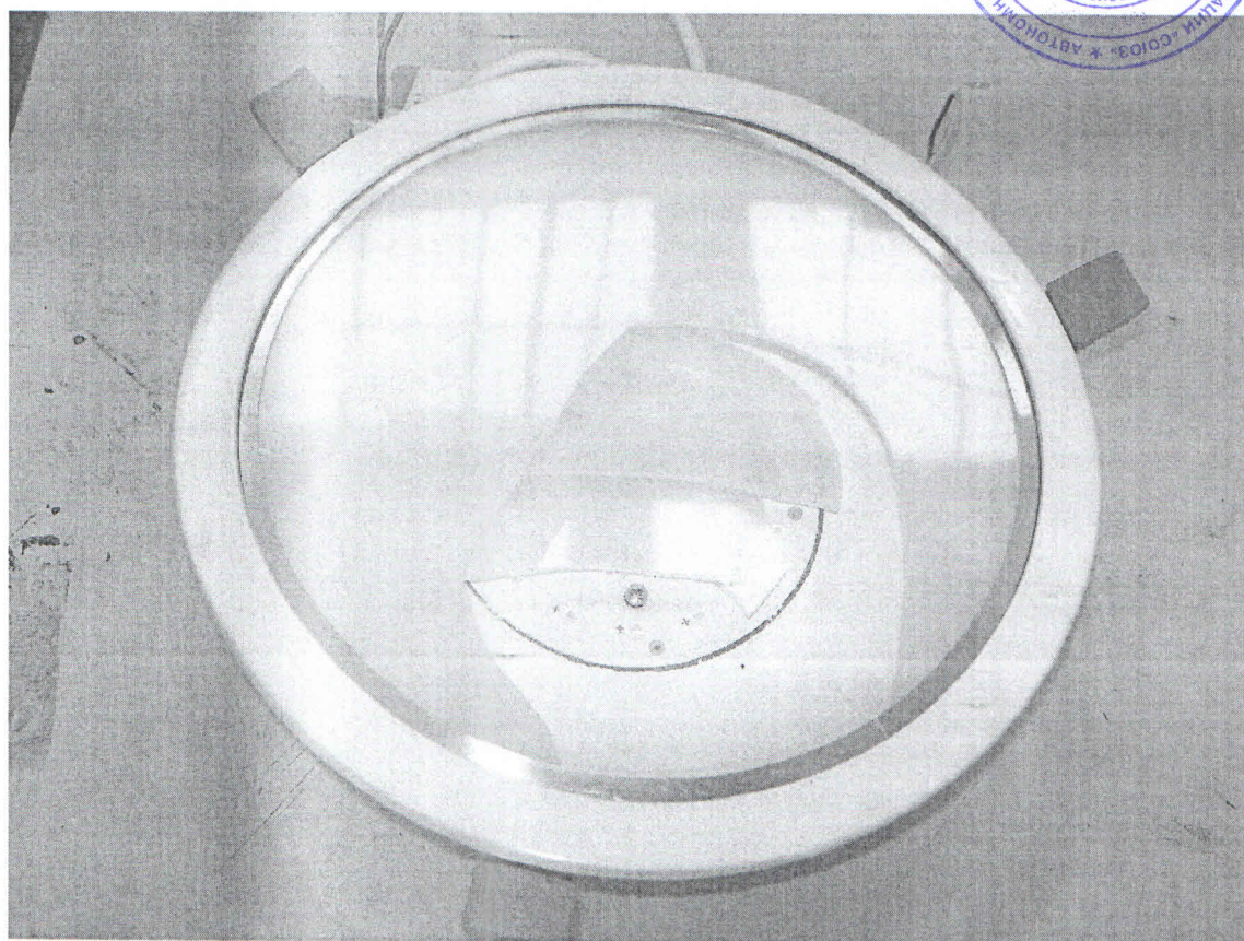
Рис. 2 Вид на наиболее слабую часть оболочки (рассеиватель) светильника после испытаний.
